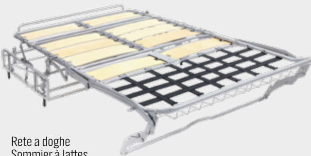
Sistema alzarete ROLLER con ruote Système à roulettes ROLLER ROLLER lift system
