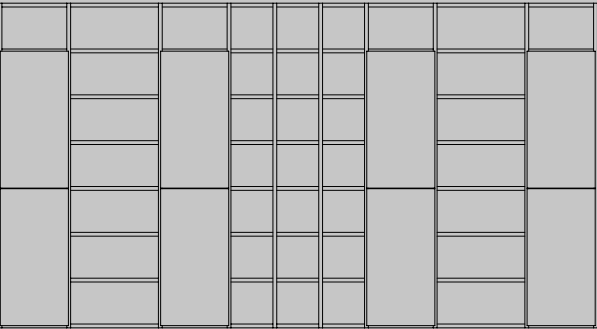
LIBRERIA SL01 Dimensions
