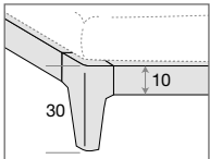
GIROLETTO LEGNO IN PANNELLO LISTELLARE RIVESTITO NOCE CANALETTO – PIEDE IN MASSELLO DI NOCE CANALETTO
