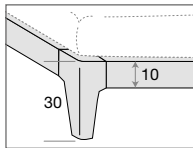
GIROLETTO LEGNO IN PANNELLO LISTELLARE RIVESTITO NOCE CANALETTO – PIEDE IN MASSELLO DI NOCE CANALETTO
