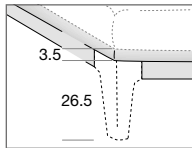
GIROLETTO LEGNO E IMBOTTITO IN PANNELLO DI LISTELLARE NOCE CANALETTO E IMBOTTITO IN GOMMAPIUMA E RIVESTITO CON TESSUTI DA CAMPIONARIO – PIEDE IN MASSELLO DI NOCE CANALETTO
