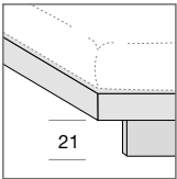
GIROLETTO FLUTTUANTE CON PIEDE IN VETRO FLOATING BED SORROUND WITH GLASS FEET
