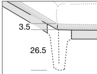
GIROLETTO LEGNO E IMBOTTITO IN PANNELLO DI LISTELLARE NOCE CANALETTO E IMBOTTITO IN GOMMAPIUMA E RIVESTITO CON TESSUTI DA CAMPIONARIO – PIEDE IN MASSELLO DI NOCE CANALETTO WOODEN BED SURROUND AND UPHOLSTERED IN CANALETTO WALNUT BLOCKBOARD PANEL AND UPHOLSTERED IN FOAM RUBBER AND COVERED WITH SAMPLE FABRICS – FOOT IN SOLID CANALETTO WALNUT
