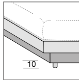
GIROLETTO FLUTTUANTE CON CONTENITORE IN METALLO. SPAZIO UTILE CONTENITORE H. 16 CM FLOATING BED SORROUND WITH METAL CONTAINER. USEFUL CONTAINER SPACE H. 16CM
