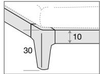
GIROLETTO LEGNO IN PANNELLO LISTELLARE RIVESTITO NOCE CANALETTO – PIEDE IN MASSELLO DI NOCE CANALETTO WOODEN BED SURROUND IN BLOCKBOARD PANEL COVERED IN CANALETTO WALNUT – FOOT IN SOLID CANALETTO WALNUT
