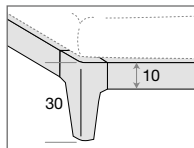
PANNELLO IMBOTTITO NON SFODERABILE UPHOLSTERED PANEL WITHOUT REMOVABLE COVER
