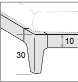
GIROLETTO LEGNO WOODEN BED SURROUND
