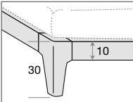
GIROLETTO LEGNO IN PANNELLO LISTELLARE RIVESTITO NOCE CANALETTO – PIEDE IN MASSELLO DI NOCE CANALETTO WOODEN BED SURROUND IN BLOCKBOARD PANEL COVERED IN CANALETTO WALNUT – FOOT IN SOLID CANALETTO WALNUT
