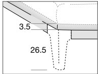
GIROLETTO LEGNO E IMBOTTITO IN PANNELLO DI LISTELLARE NOCE CANALETTO E IMBOTTITO IN GOMMAPIUMA E RIVESTITO CON TESSUTI DA CAMPIONARIO – PIEDE IN MASSELLO DI NOCE CANALETTO WOODEN BED SURROUND AND UPHOLSTERED IN CANALETTO WALNUT BLOCKBOARD PANEL AND UPHOLSTERED IN FOAM RUBBER AND COVERED WITH SAMPLE FABRICS – FOOT IN SOLID CANALETTO WALNUT
